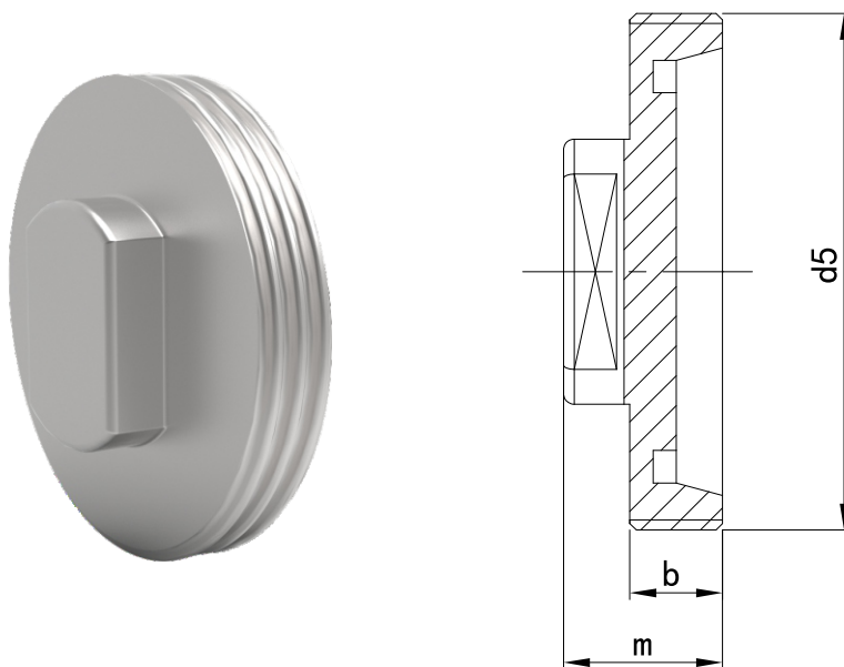
DIN11851 由任牙接头盲板C 316L Union Blind
