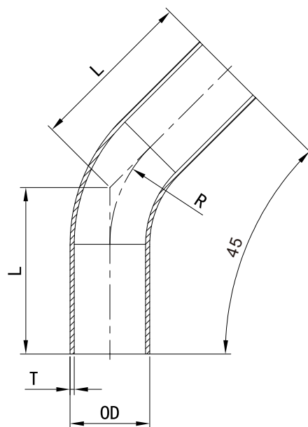
DIN11865 45°弯头 长焊 C系列 Automatic Weld: 45° Elbow 304L
