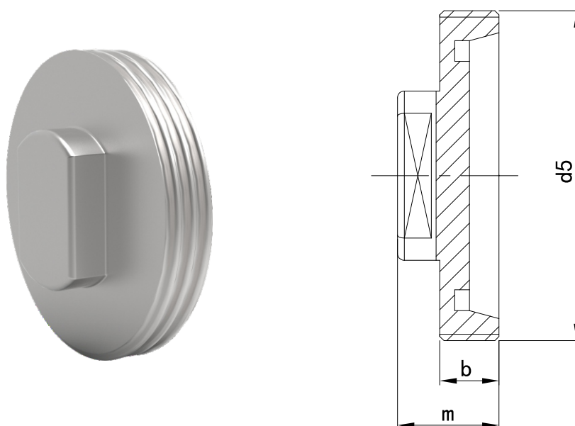
DIN11851 由任牙接头盲板C 304L Union Blind
