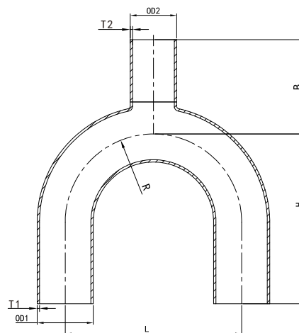
DIN11865 焊式U型三通 C系列 304L Automatic Weld 180° Return-Bend Reducing Tee //
