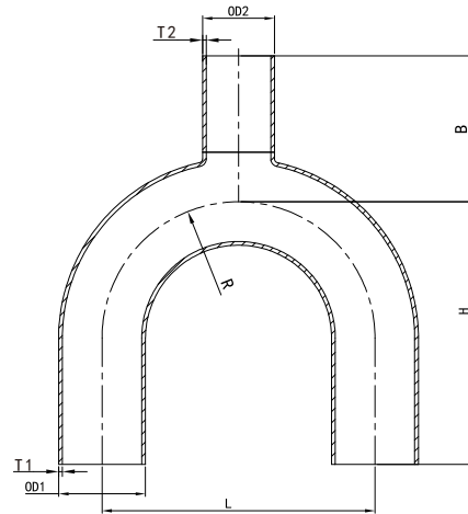
DIN11865 焊式U型三通 C系列 316L Automatic Weld 180° Return-Bend Reducing Tee //
