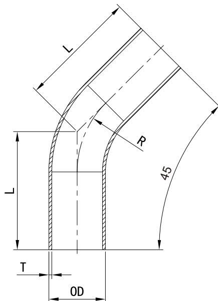
DIN11865 45°弯头 长焊 C系列 Automatic Weld: 45° Elbow 316L
