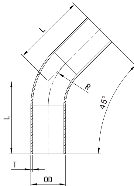
DIN11852 45°弯头 长焊 Automatic Weld: 45° Elbow 304L
