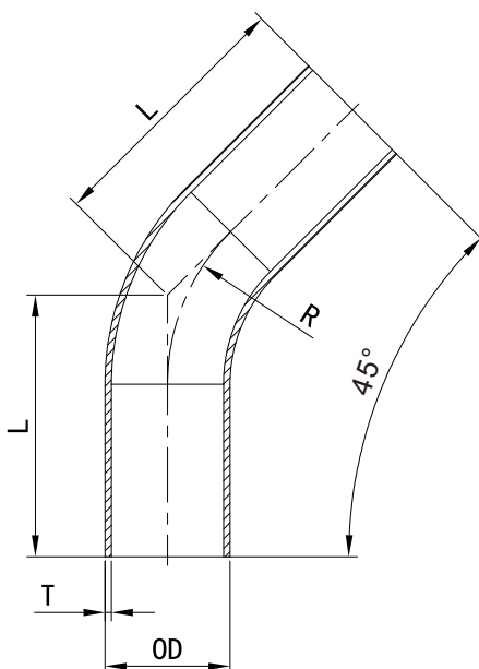
DIN11852 45°弯头 长焊 Automatic Weld: 45° Elbow 316L
